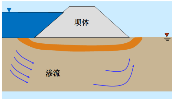
图 5 渗透破坏之管涌
